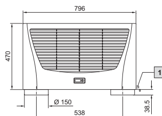
1 Kondensavledning 1/2", flexibel
