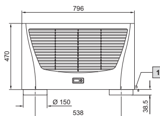
1 Tuyau flexible d'écoulement des condensats 1/2"
