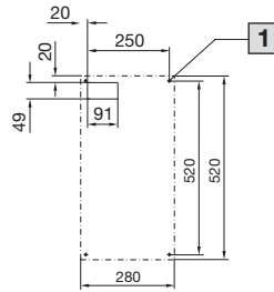
Montageudskæring til indbygning
