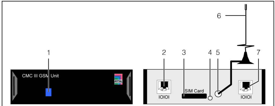
Abb./Fig./Fig. 3: Anzeigeelemente, Stecker und Anschlüsse / Display elements, plugs and connectors / Organes de signalisation, fiches et raccords
