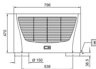
1 冷凝水排放 1/2", 柔性
