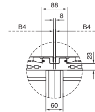
Detalj Y (kun ved SE 5842.500 og SE 5846.500)
