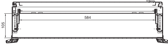
Kesit B - B
