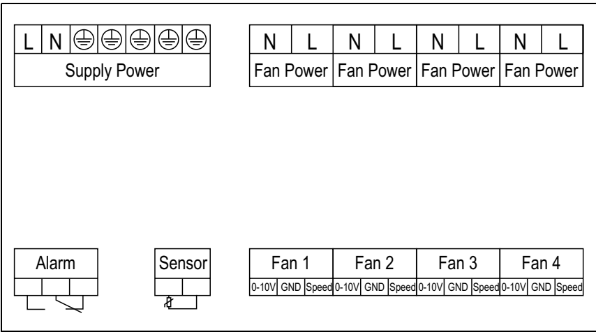
Fig. 2: Allacciamento elettrico
