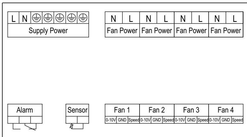
図 2: 電気接続図
