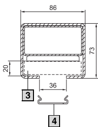
Schnitt A – A
