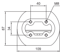
Anschlussplatte oben
