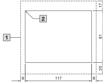
Montageausschnitt
