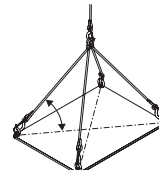
Seilzug Der zwischen Dachblech und Seil vorhandene Seilzugwinkel beeinflusst in starkem Maße die zulässige Gesamtbelastung. Der Seilzugwinkel darf nicht kleiner als 45° sein und sollte nach Möglichkeit nicht unter 60° liegen.
