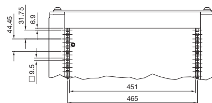
Detalle Y
