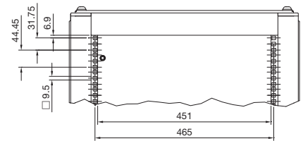
Detalhe Y
