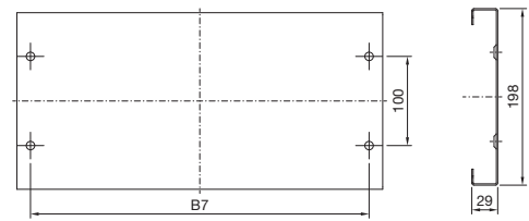
Pantallas de zócalo, ciegas, 200 mm de altura Vista frontal
