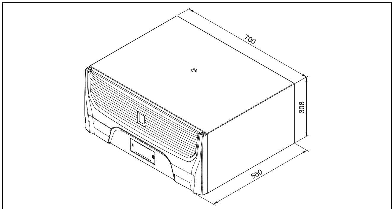
Bild 30: Mått SK 3185730
