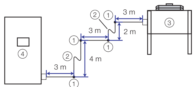
Abb. 20: Vereinfachte Darstellung der Anschlussleitungen
