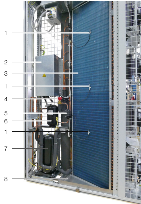
Abb. 5: Kältemittelkreislauf
