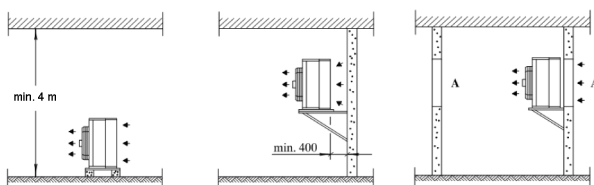
Abb. 16: Aufstellmöglichkeiten bei horizontalem Luftauslass
