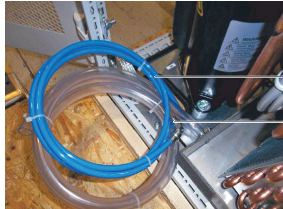
Abb. 45: Anschlussschlauch mit Anschlussstück 1/8" Außengewinde
