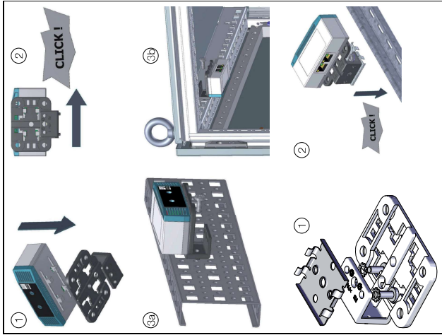
Abb./Fig./Fig. 2: Montage / Mounting / Montage
