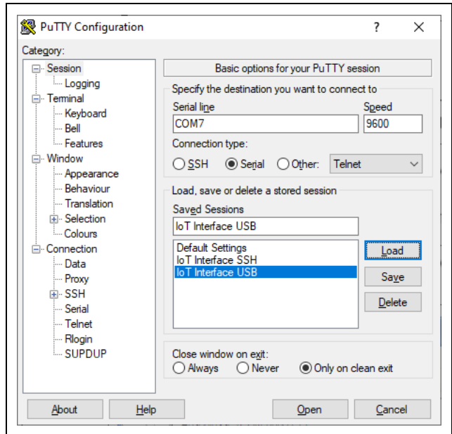
Fig. 16 : réglage de la liaison « CMC III PU USB »
