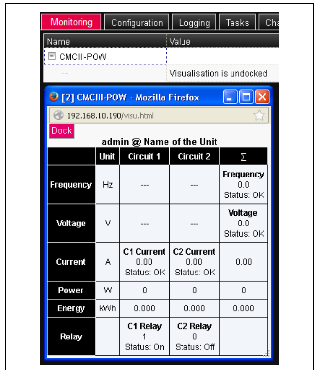
Fig. 29 : fenêtre transférée de la Power Unit
