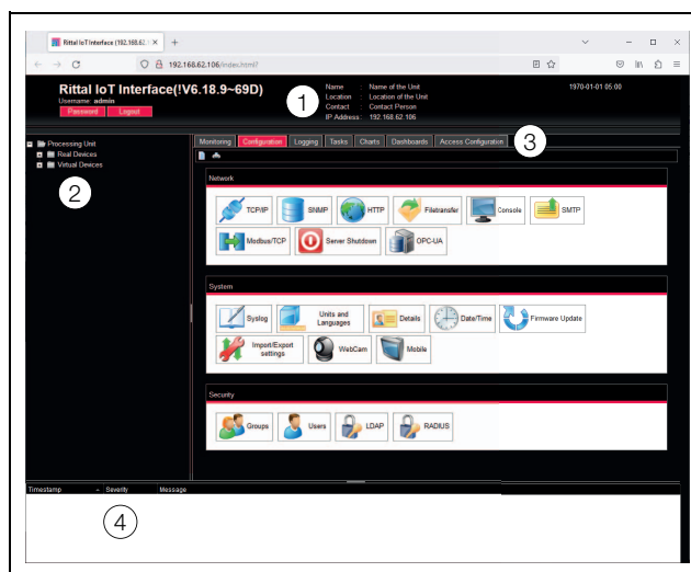
Fig. 20 : conception de l'arborescence des écrans
