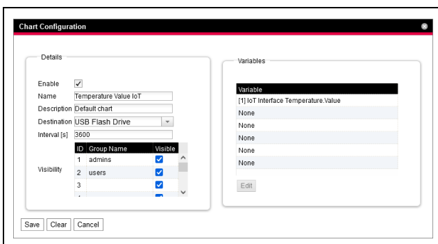
Fig. 38 : dialogue « Chart Configuration »
