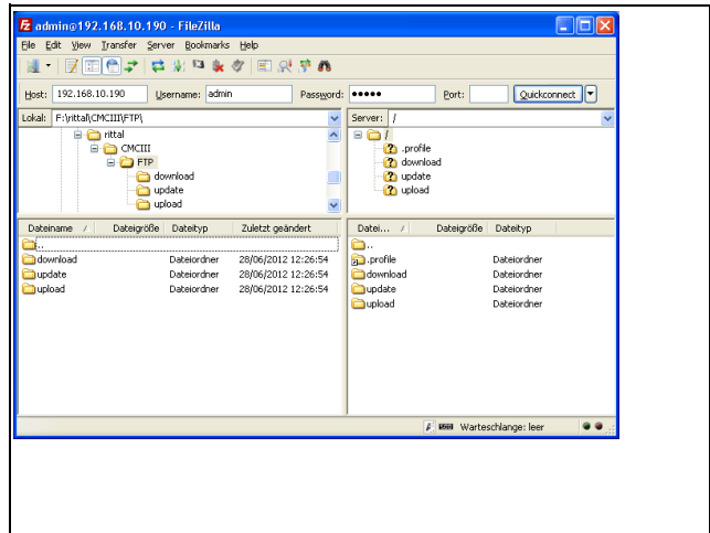
Fig. 43 : FileZilla
