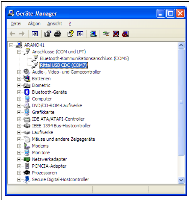
Fig. 15 : gestionnaire d'appareils
