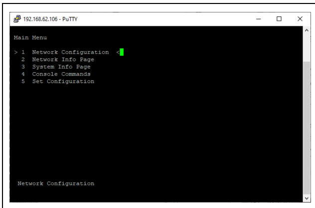
Fig. 18 : menu principal
