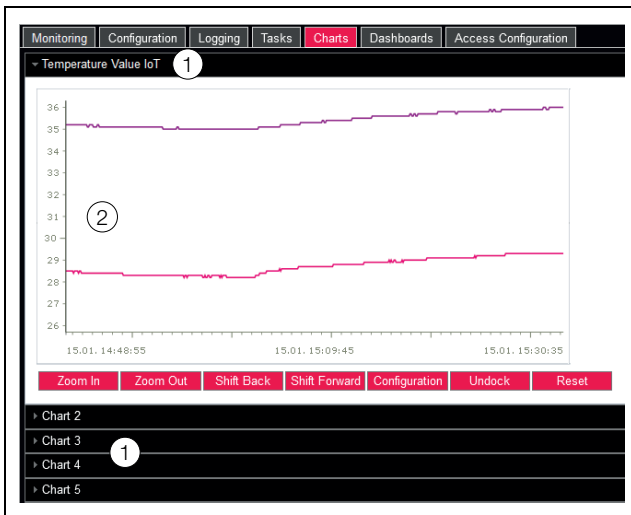
Fig. 37 : onglet Charts
