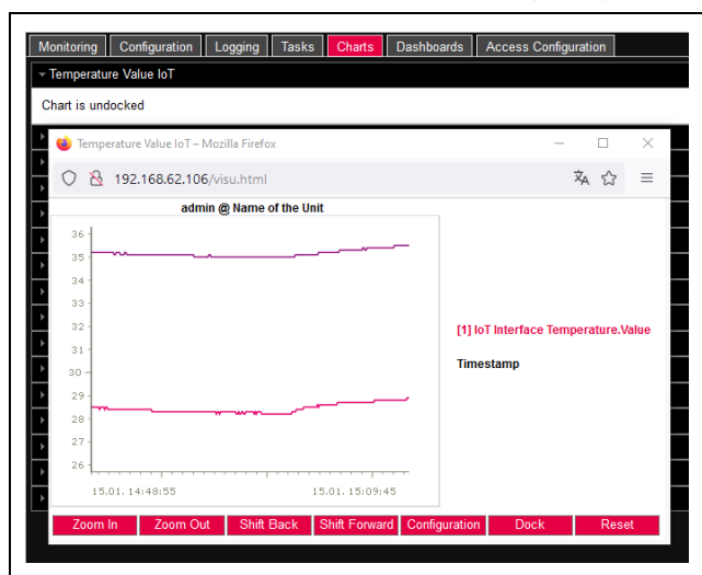
Fig. 39 : diagramme déplacé
