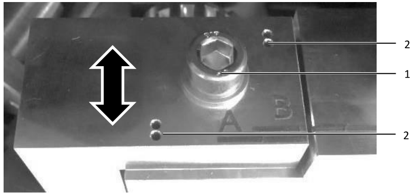
Fig. 12 : réglage de la cale d'ouverture (réglé : B)
