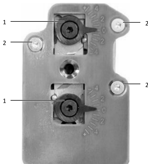
Fig. 25 : unité à dénuder
