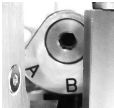
Fig. 9: réglage de la butée d'embout
