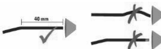
Fig. 14 : introduire correctement le câble
