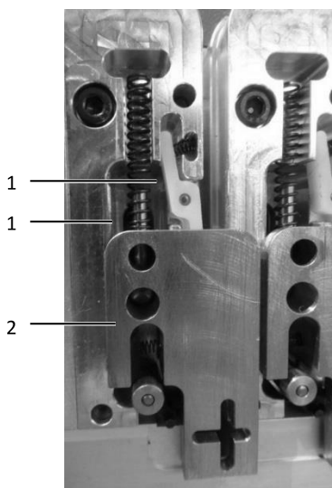
Fig. 23 : unité de transport
