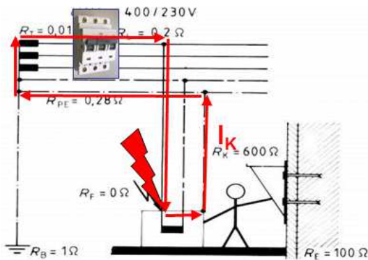
Abbildung 4: Prinzip der Abschaltung
