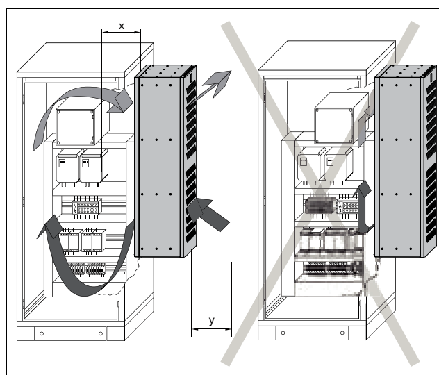
Afb. 6: Luchtcirculatie in de kast
