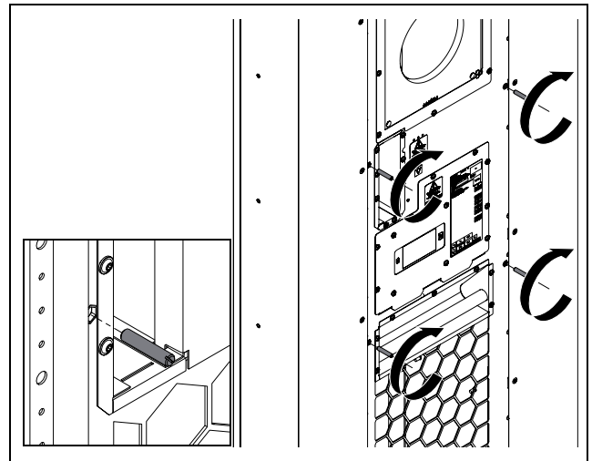
Afb. 17: Aanbrengen van de middelste draadstiften
