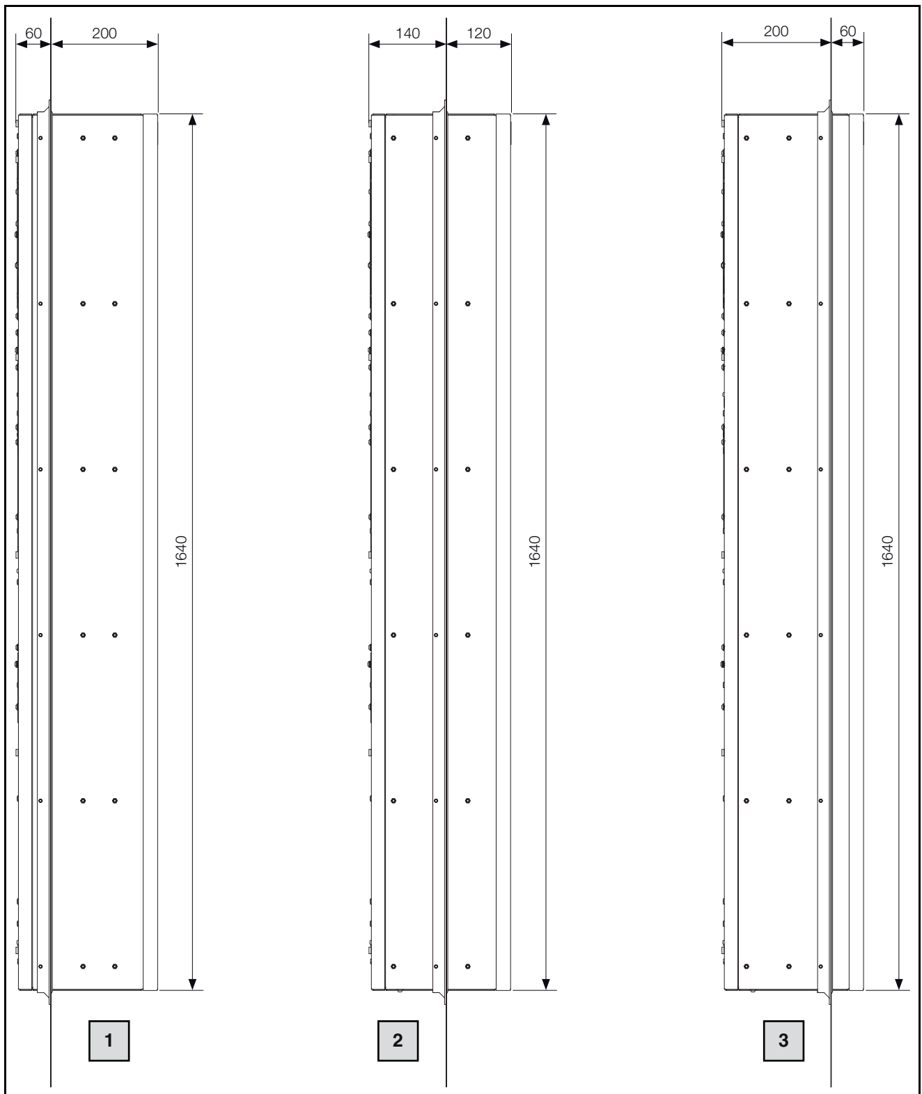
Afb. 54: Afmetingen
