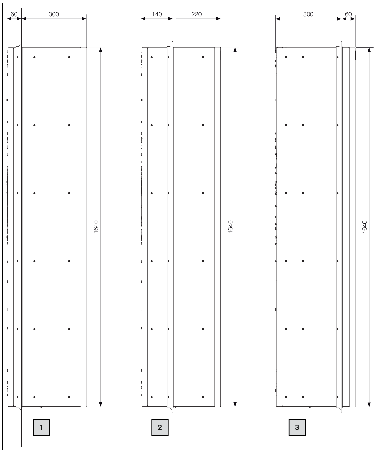
Afb. 55: Afmetingen
