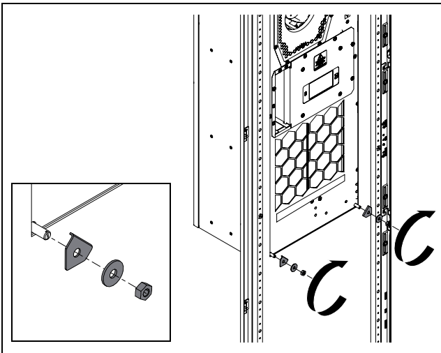
Afb. 15: Monteren van de onderste hoeksteunen
