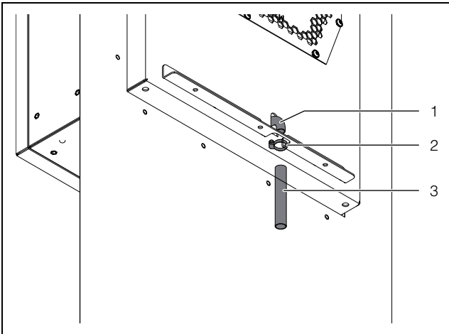
Afb. 30: Aansluiting voor condensafvoerslang
