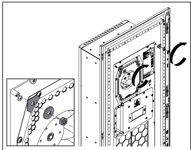
Afb. 14: Monteren van de bovenste hoeksteunen
