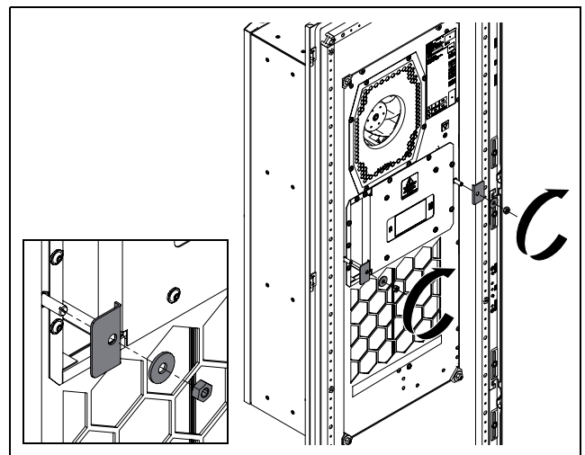
Afb. 18: Aanbrengen van de middelste L-beugels
