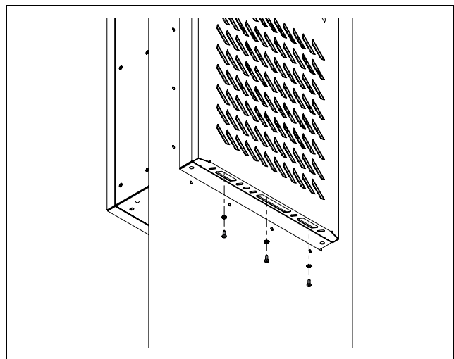
Afb. 47: Losdraaien van de bevestigingsschroeven
