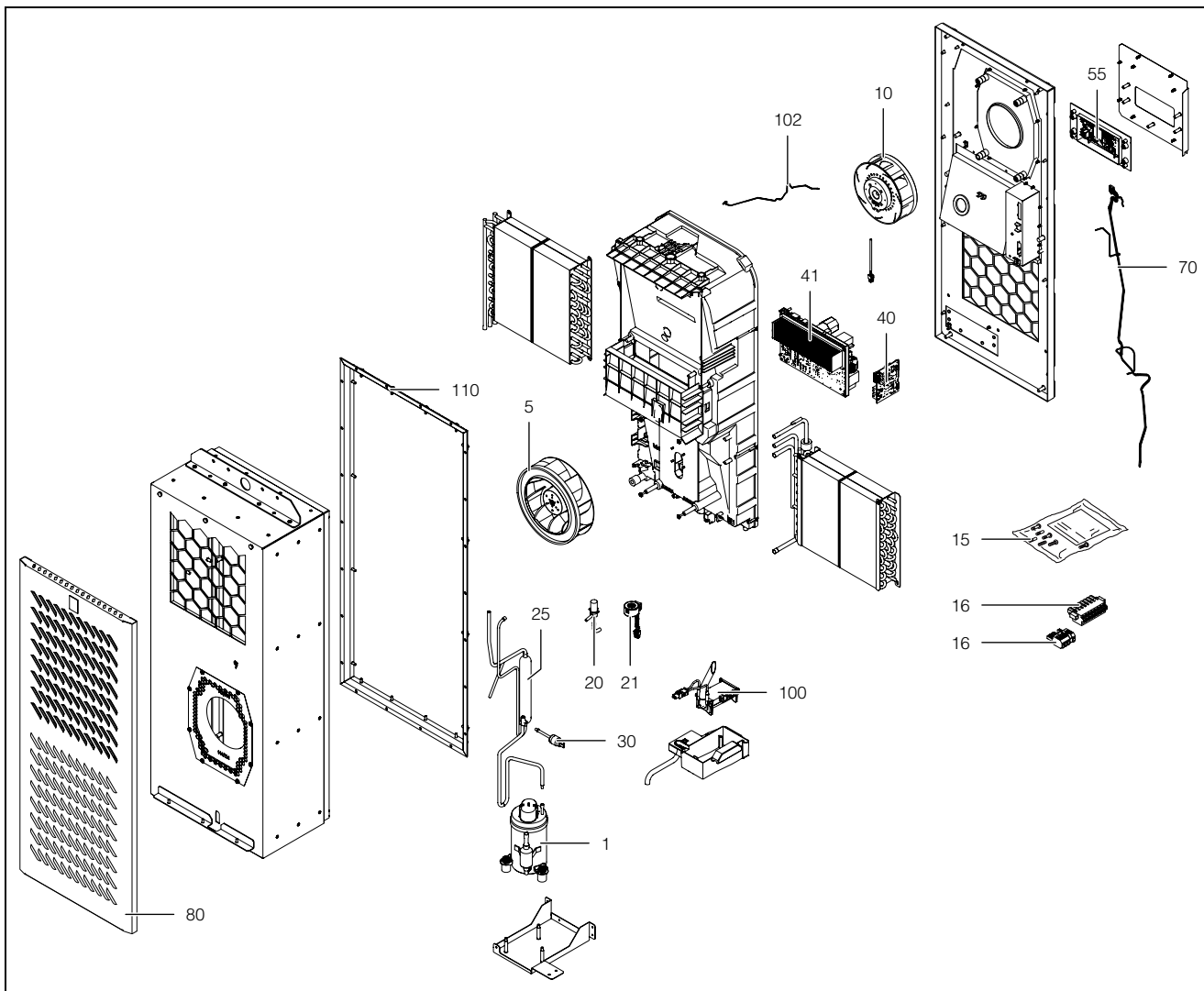
Afb. 50: Reservedelen (voorbeeldweergave)
