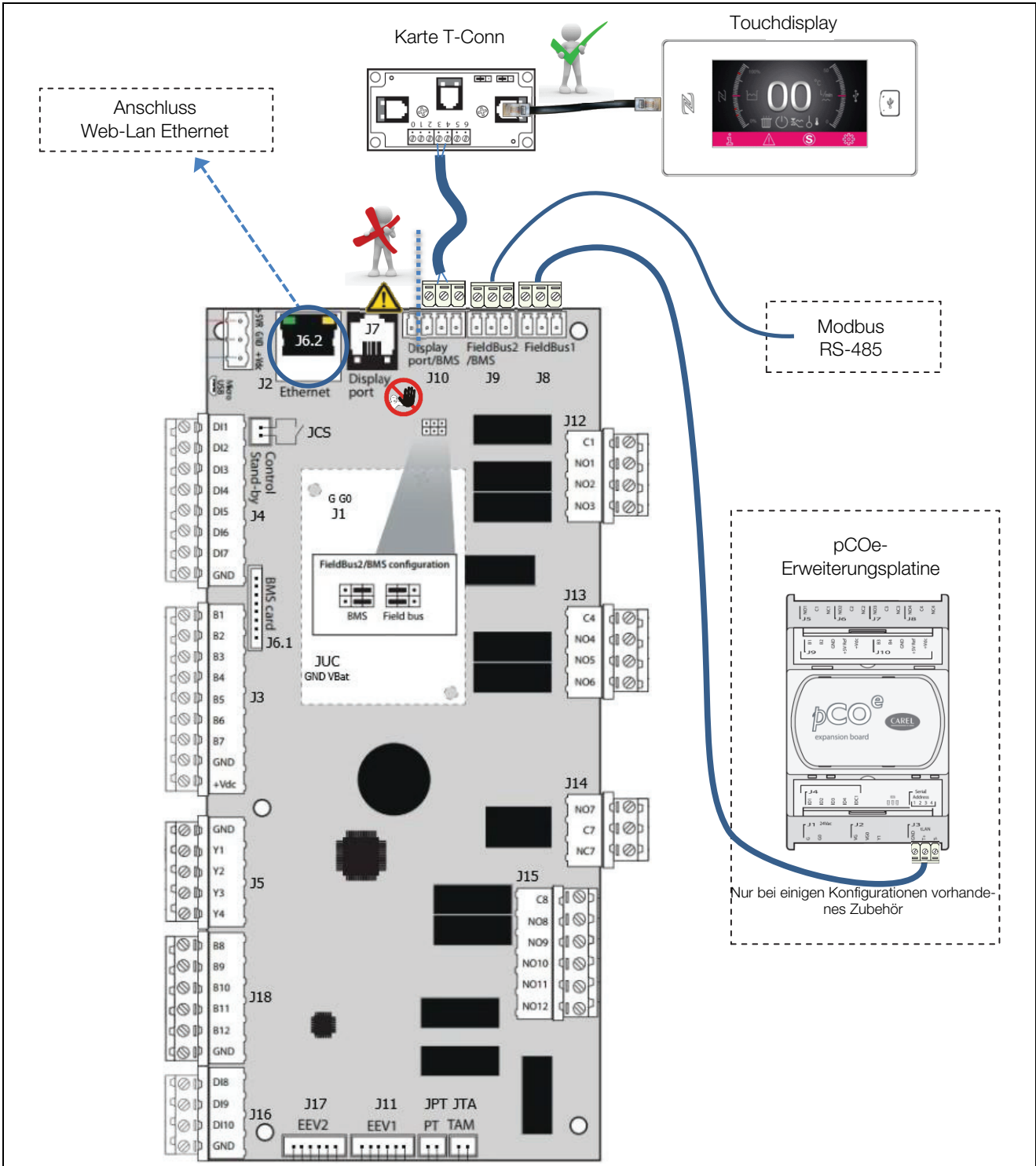
Abb. 34: Blockdiagramm
