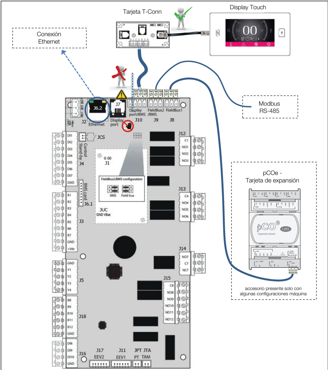
Imagen 34: Diagrama de bloques
