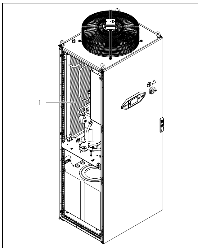
Imagen 23: Limpiar el condensador
