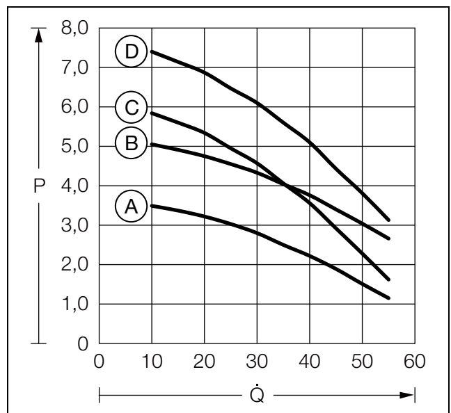
Imagen 4: Diagramas SK 3335930, SK 3335940 y SK 3335950
