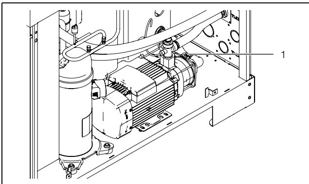
Imagen 13: Purgado de la bomba del medio refrigerante
