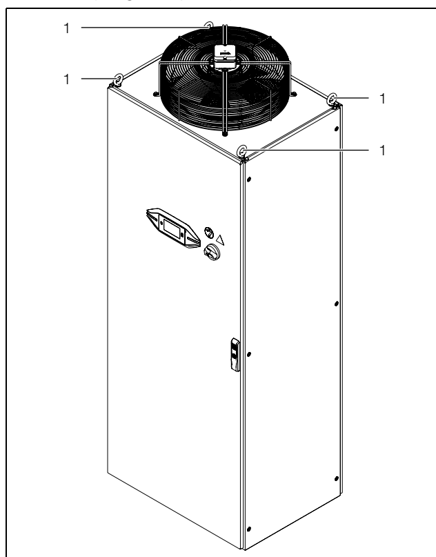
Imagen 6: Transporte
