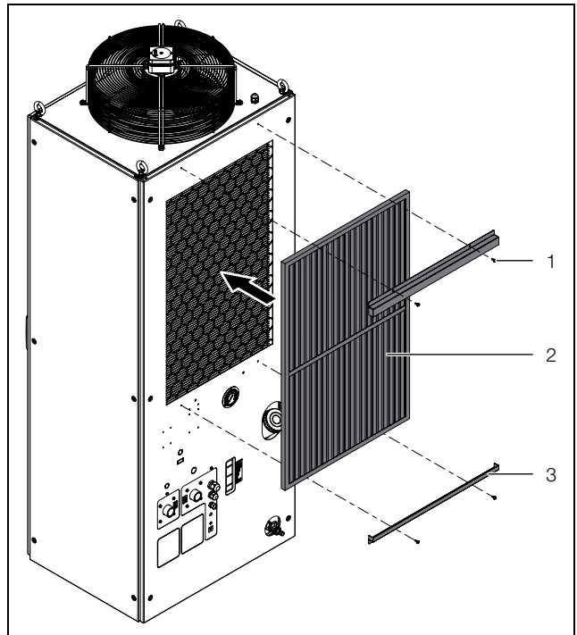
Imagen 11: Montaje de los filtros metálicos
