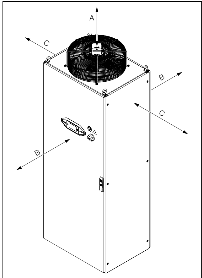
Imagen 7: Distancias mínimas
