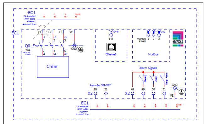
Imagen 8: Diagrama de circuitos
