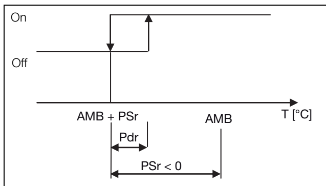
Imagen 18: Tipo de ajuste «relativo con valores límite»
