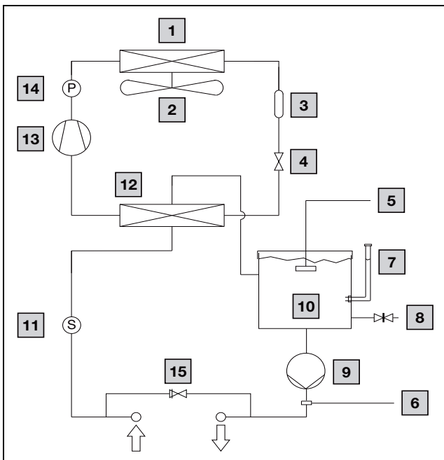
Imagen 3: Circuito del medio refrigerante (SK 33359x0)
