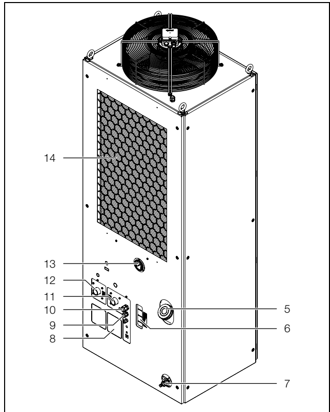
Imagen 2: Vista posterior
