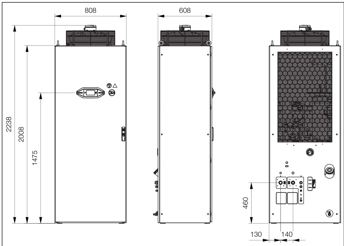
Imagen 36: Esquemas componentes
