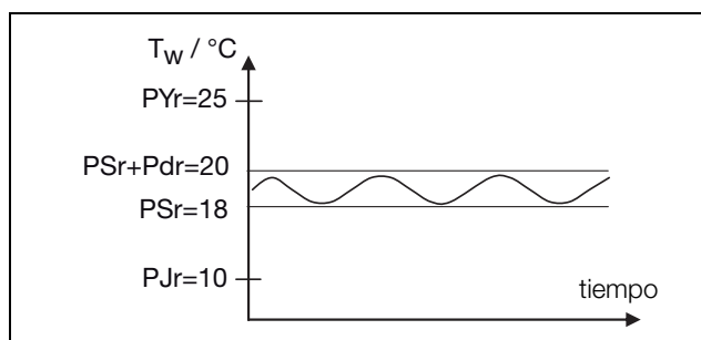
Imagen 16: Regulación «valor fijo»
