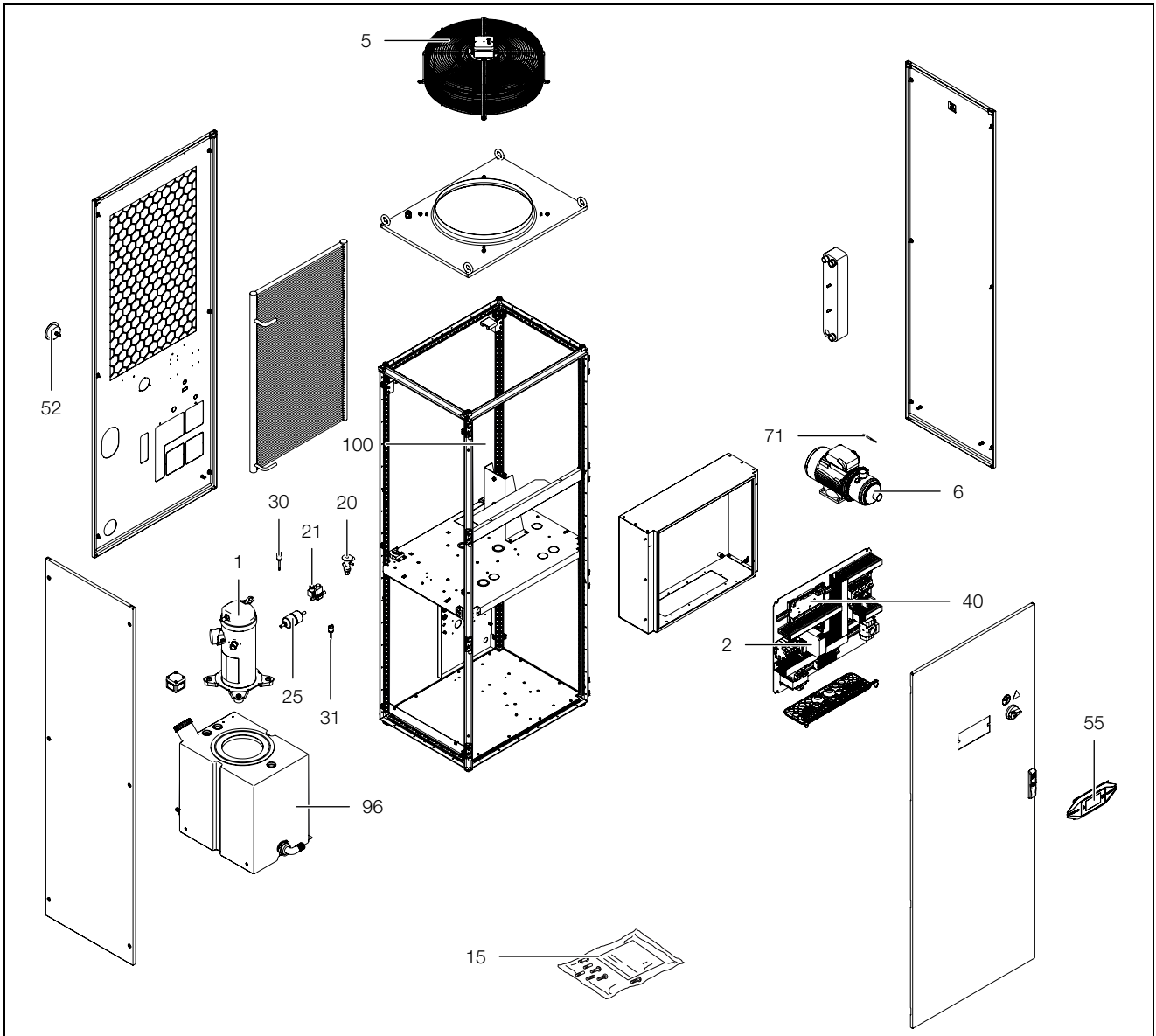
Imagen 35: Dibujo recambios
