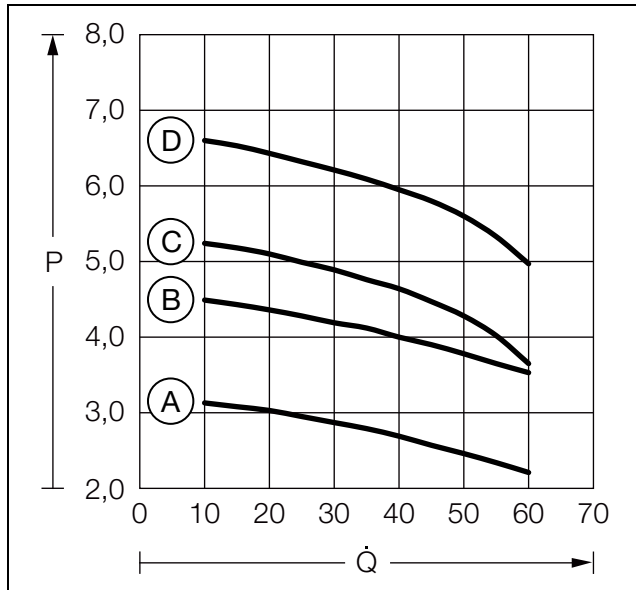
Imagen 5: Diagramas SK 3335960
