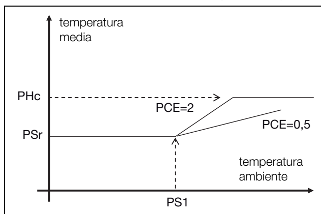
Imagen 17: Tipo de ajuste «relativo con valores límite»
