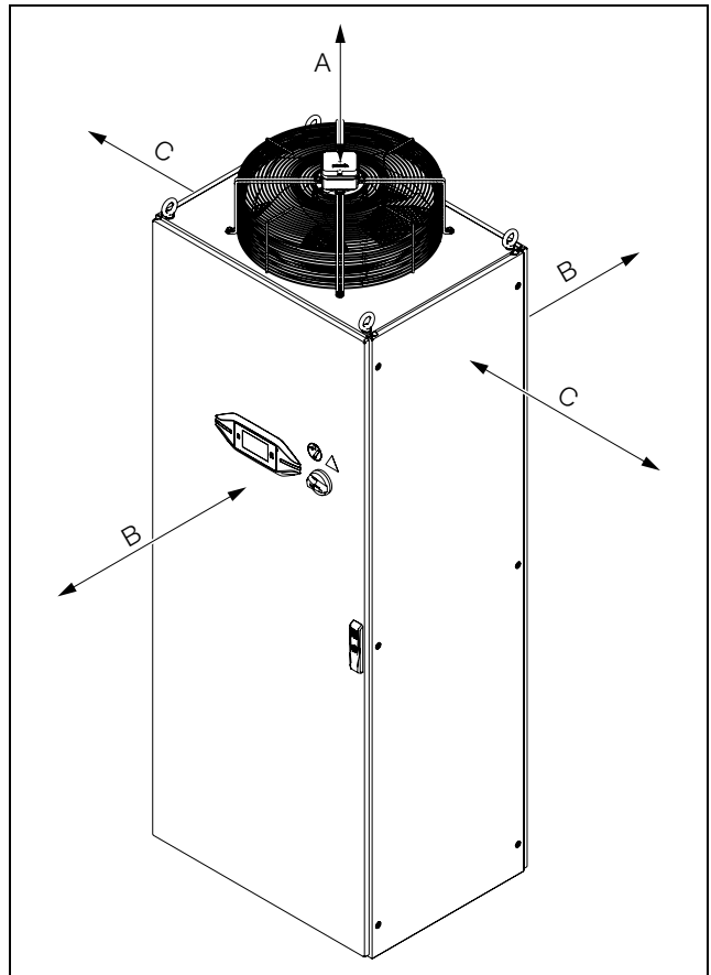
Imagen 7: Distancias mínimas
