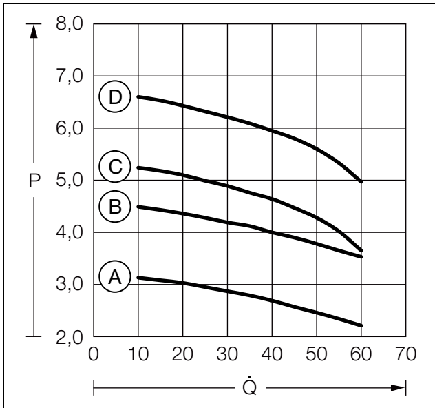
Imagen 5: Diagramas SK 3335960
