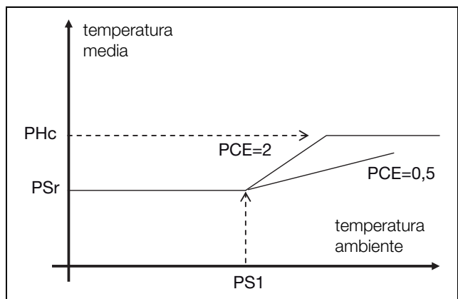
Imagen 17: Tipo de ajuste «relativo con valores límite»
