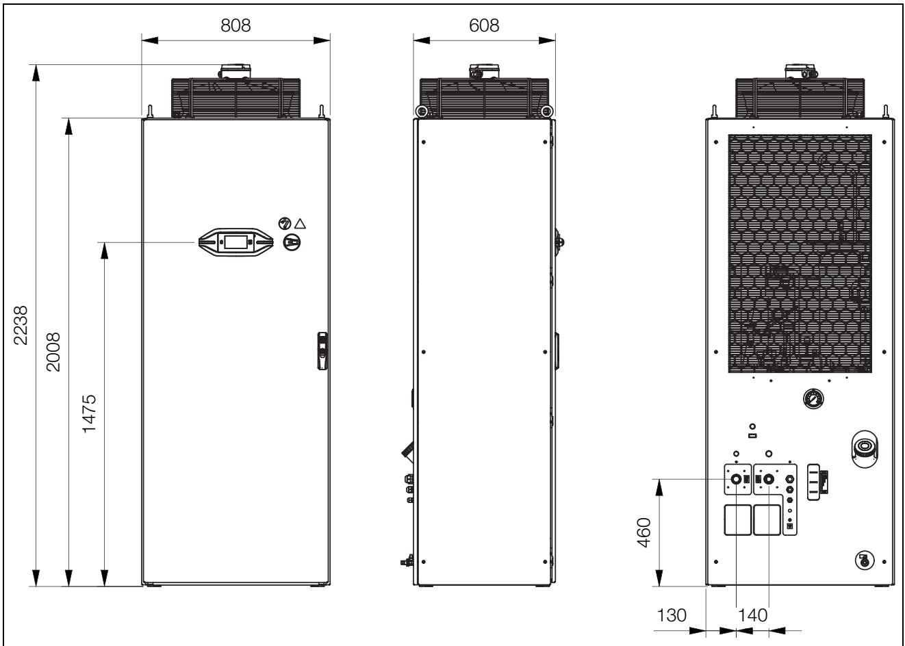
Imagen 36: Esquemas componentes
