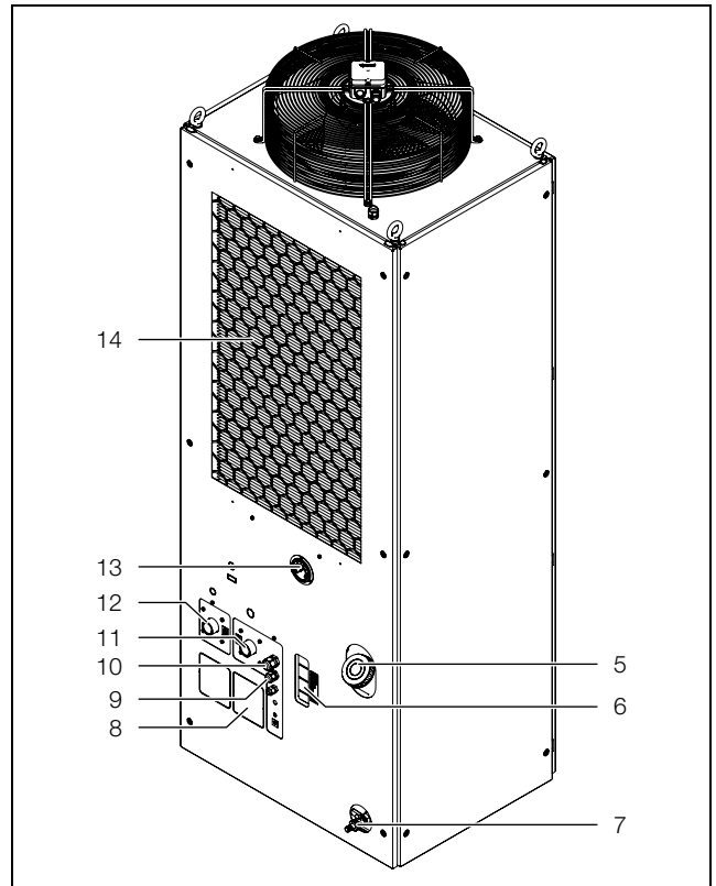
Imagen 2: Vista posterior
