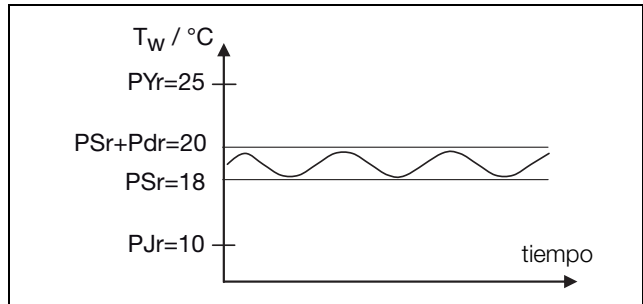
Imagen 16: Regulación «valor fijo»
