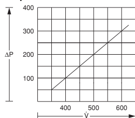
Характеристика гидравлического сопротивления SK 3247.000
