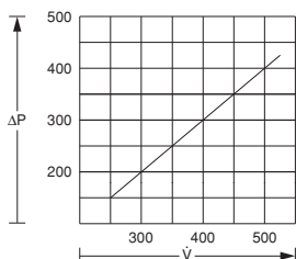
Характеристика гидравлического сопротивления SK 3218.100
