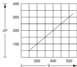
Характеристика гидравлического сопротивления SK 3217.100
