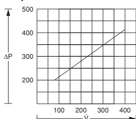
Характеристика гидравлического сопротивления SK 3249.100
