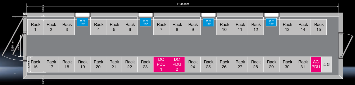
40ft 일체형 냉각(16kW 냉각) 2.4W x 12L x 2.9H m
