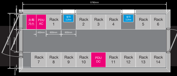
40ft 분리형 냉각(30kW 냉각) 2.4W x 12L x 2.9H m
