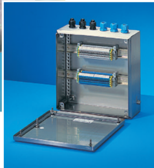
Monteren van aansluitklemmen en kabelwartels standaard en explosieveilig
