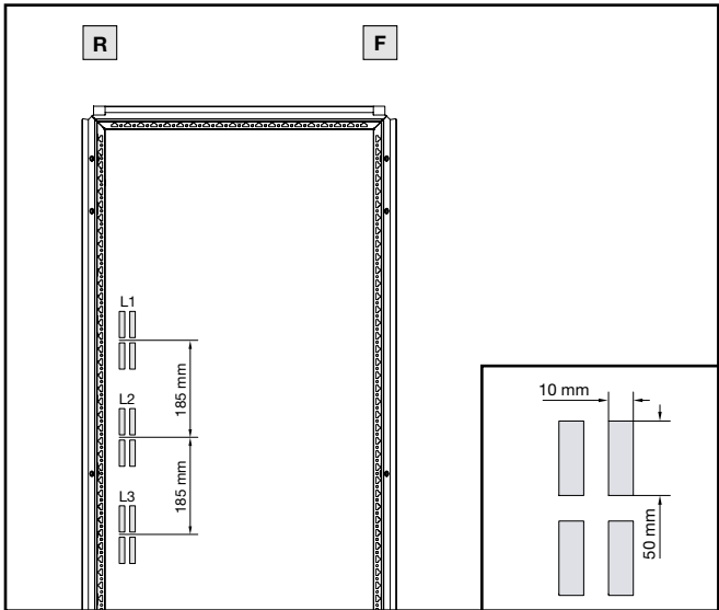
Bestückung Sammelschienenhalter 50 x 10 Rückbereich
