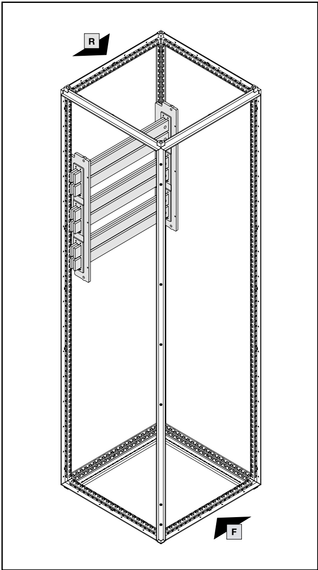
Bestückung Sammelschienenhalter 50 x 10 Rückbereich
