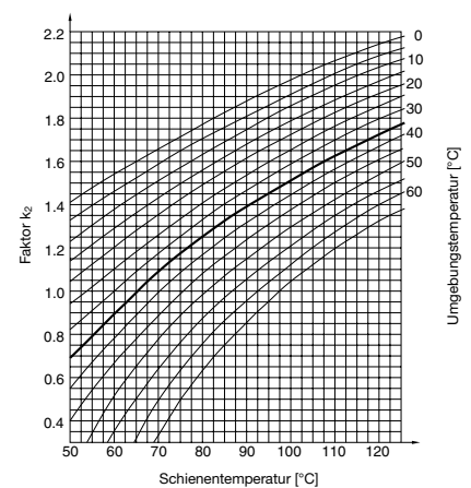
Korrekturfaktordiagramm nach DIN 43 671
