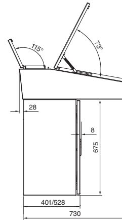
Oppbygging 2-delt
